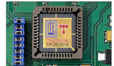
Scalony wielokanałowy układ odczytowy do tranzystorowych detektorów THz (AMS 350nm)
