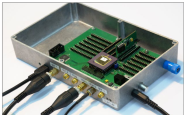
Środowisko testowe scalonego układu odczytowego licznika cząstek
