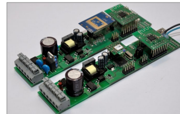
Sterownik inteligentnej oprawy oświetleniowej oraz moduł mostka ZigBee – Bluetooth
